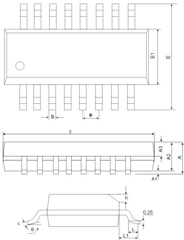
图 10：封装尺寸
