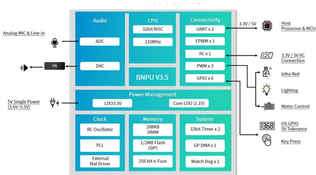
图 1: CI13162 功能框图
